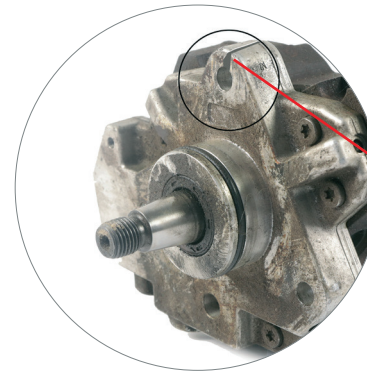
Gehäuse gebrochen housing broken
